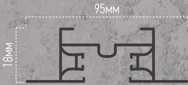
СЕЧЕНИЕ ШИНОПРОВОДА СЕРИИ TOP-LINE
