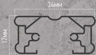
СЕЧЕНИЕ ШИНОПРОВОДА СЕРИИ TOP-LINE
